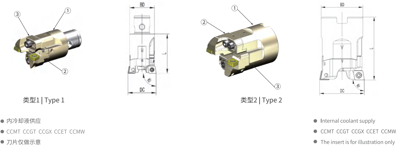
技术参数 | Technical parameters
