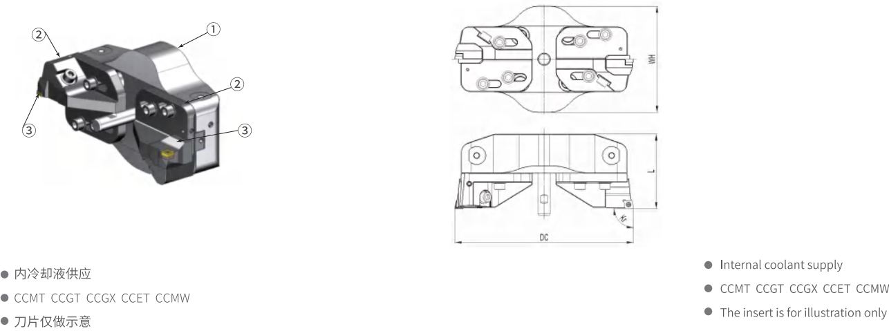
技术参数 | Technical parameters 单位 | Unit: mm
